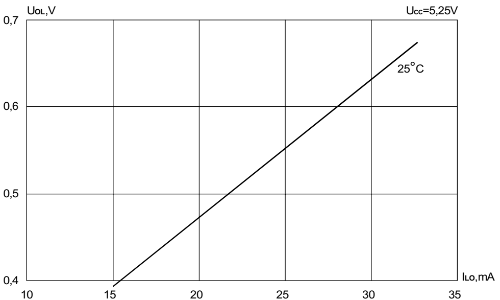
Зависимость U_{OL}=f(I_{OL}) на выводах 14-19, 21, 22
