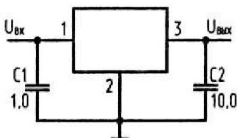
Типовая схема включения КР1158ЕН12
