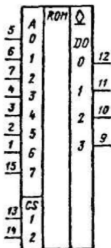
Условное графическое обозначение К155РЕ21
