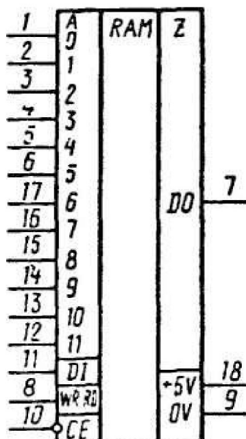
Условное графическое обозначение КР132РУ5, КМ132РУ5
