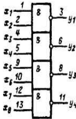
Условное графическое обозначение К158ЛА3
