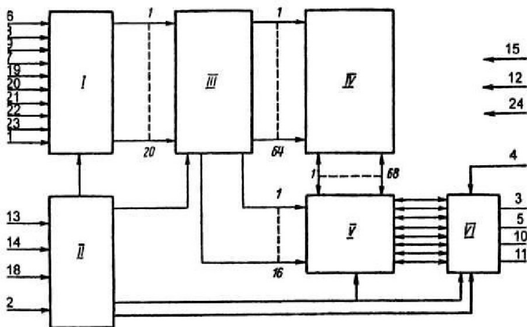
Структурная схема КР1601РР1:
