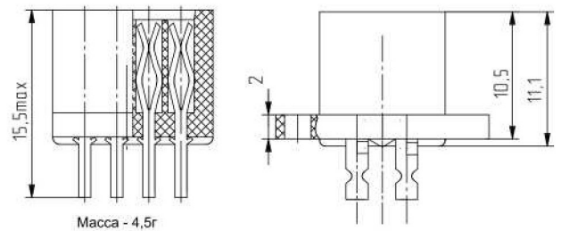
Рисунок 12 Розетка РГ1Н-1-7
